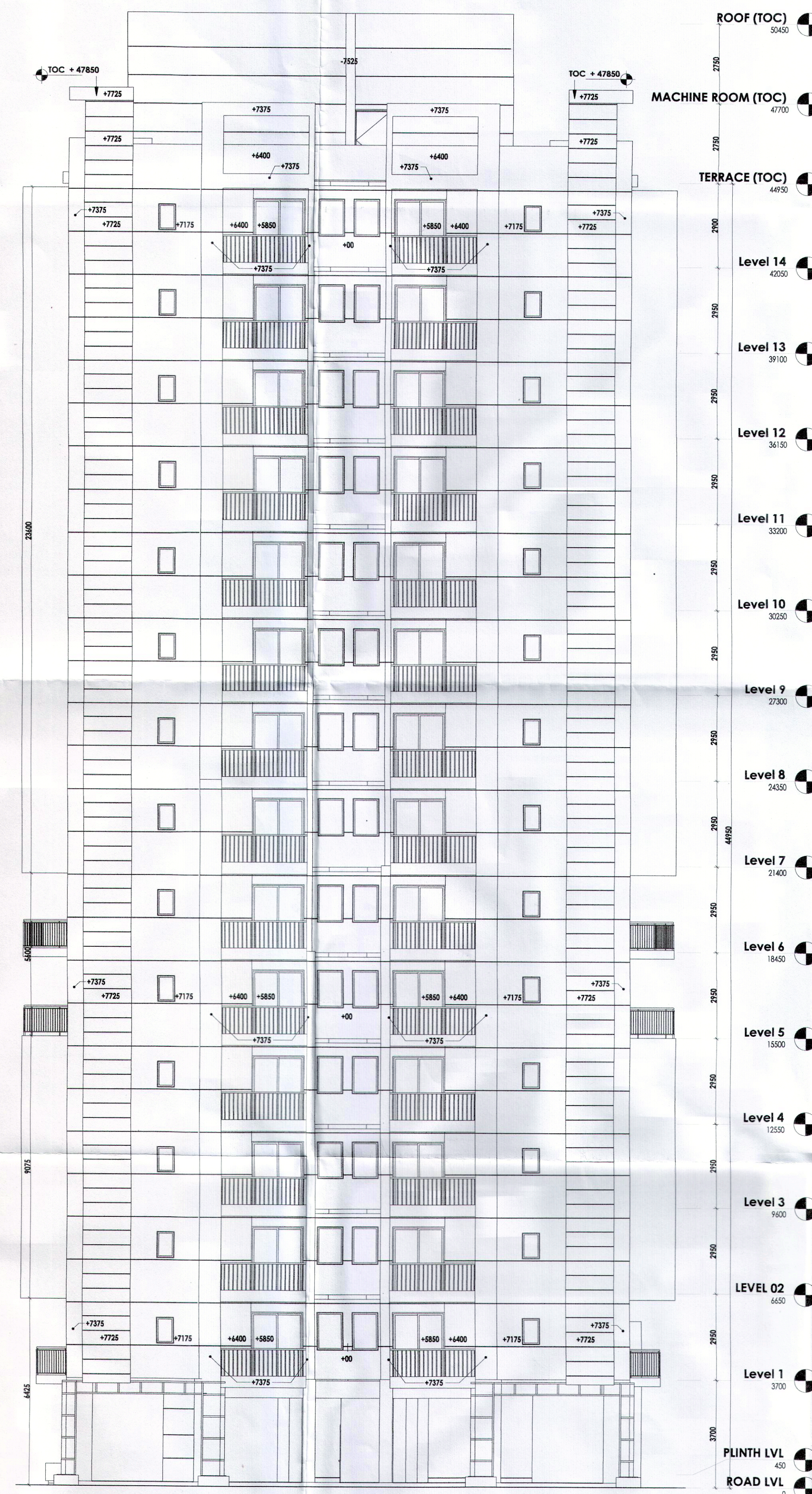
ELEVATION - D
