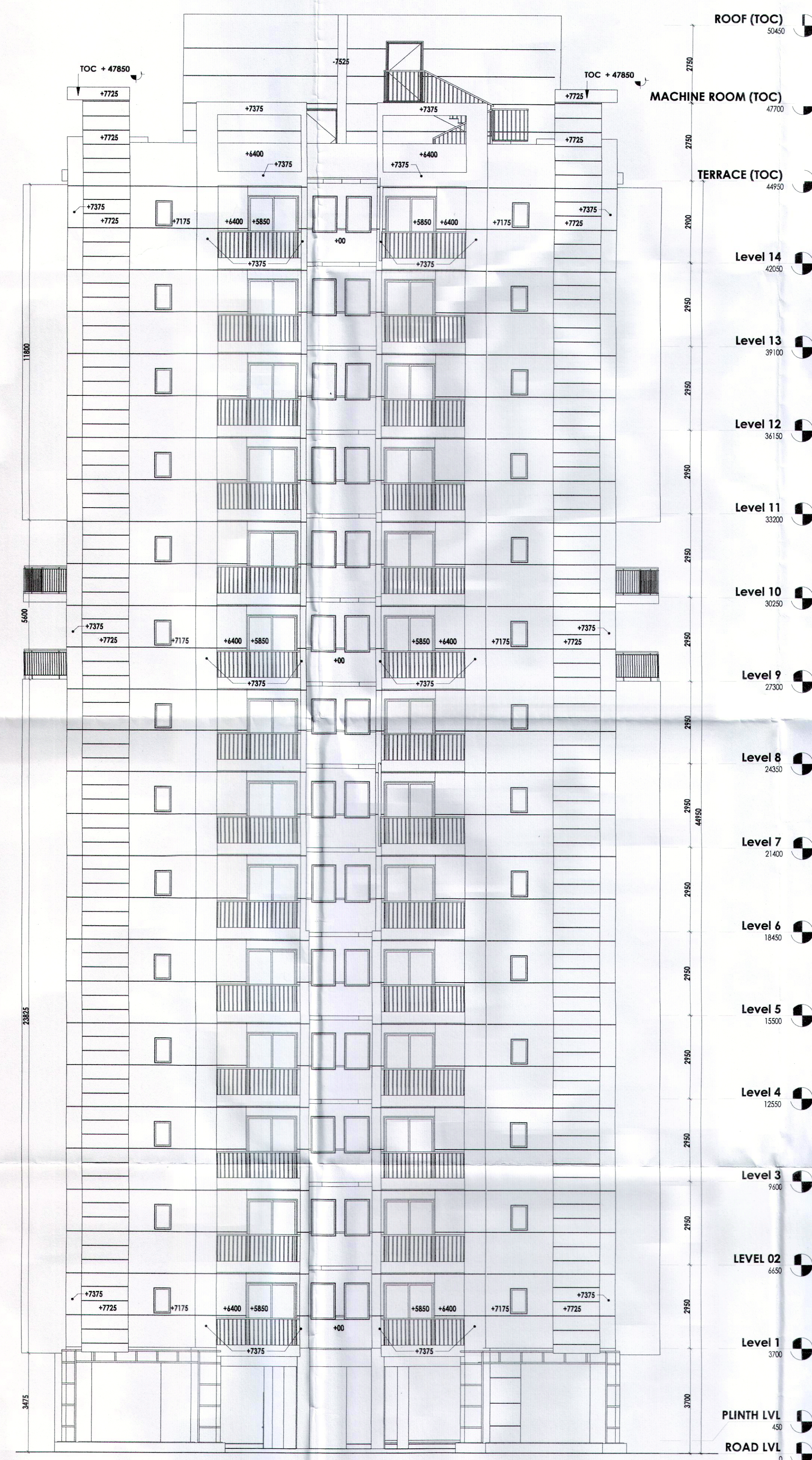
ELEVATION - B
